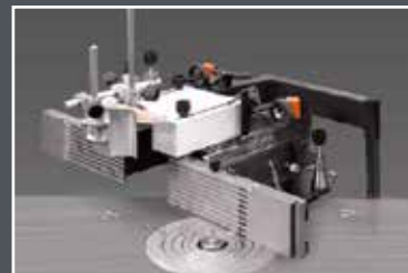
► Automata csapozó védőburkolat
